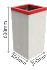
Nk 2003 SIMPLE - 50 LITROS
